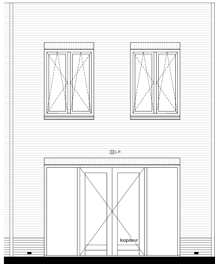
achtergevel
