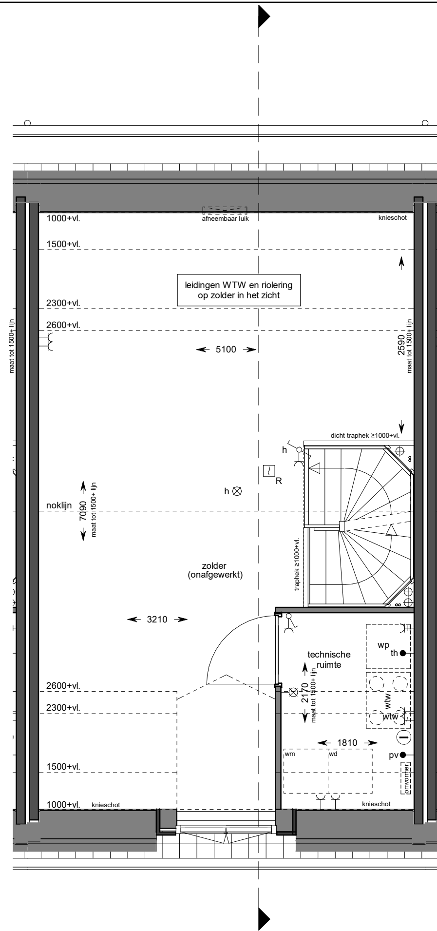
tweede verdieping
