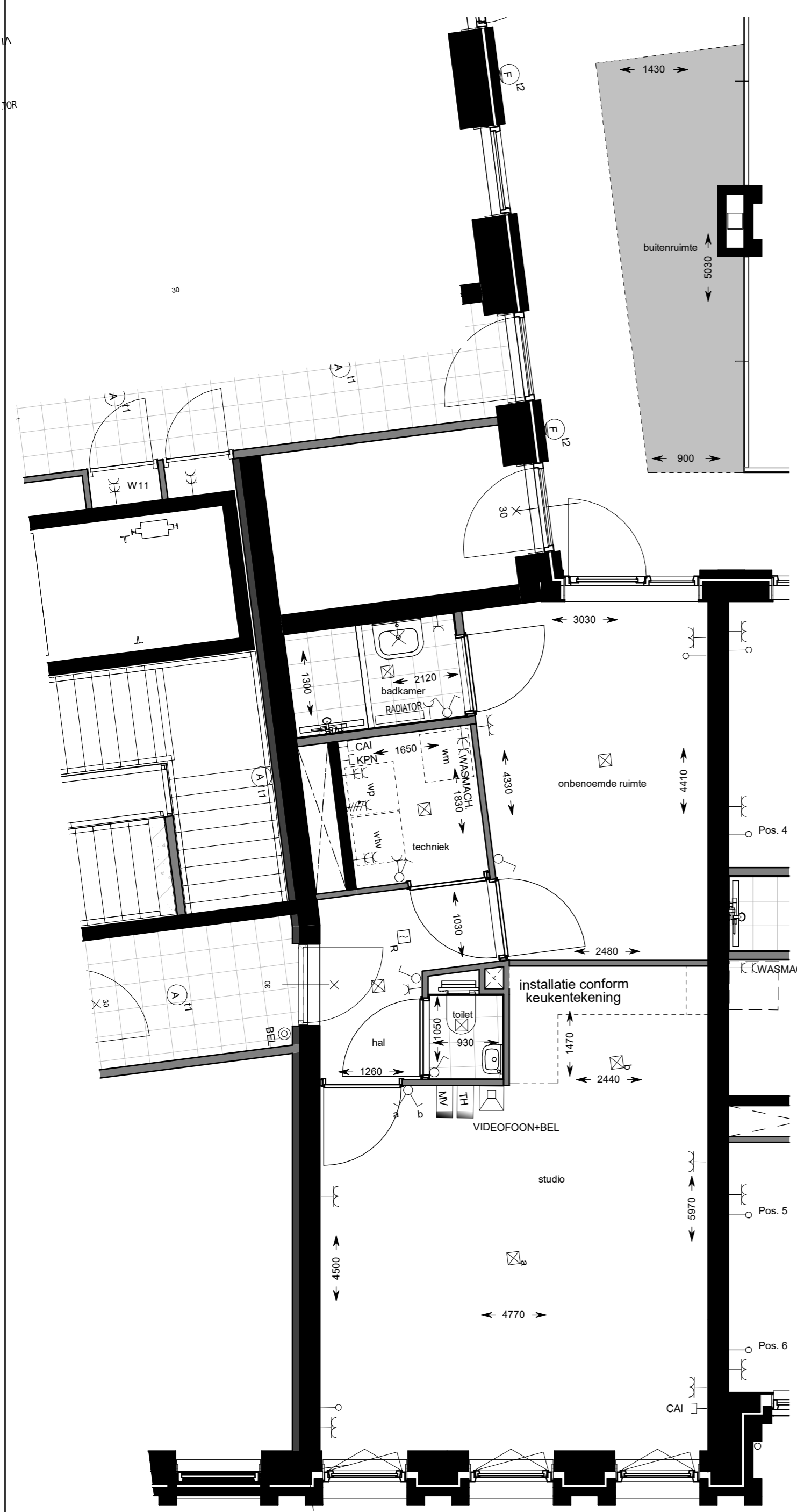
eerste verdieping
