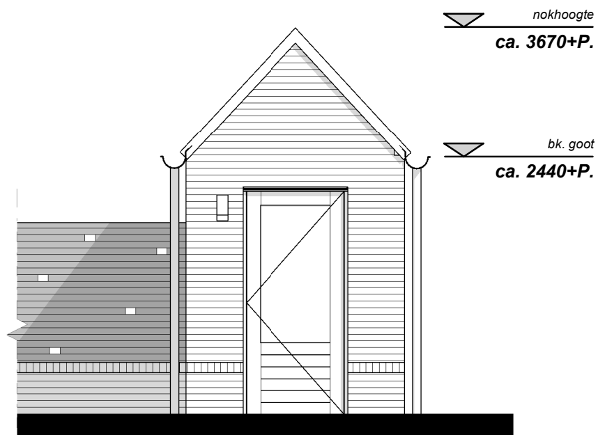
voorgevel
