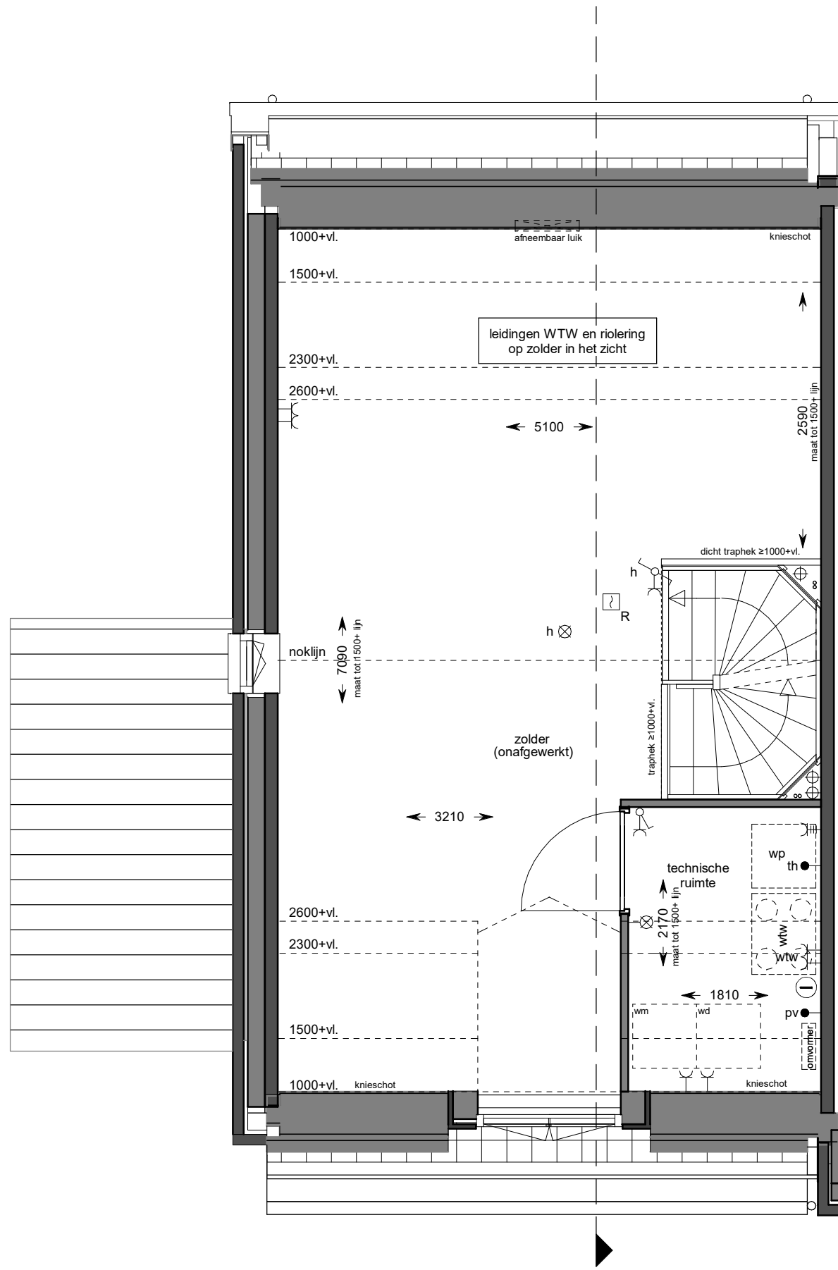
tweede verdieping
