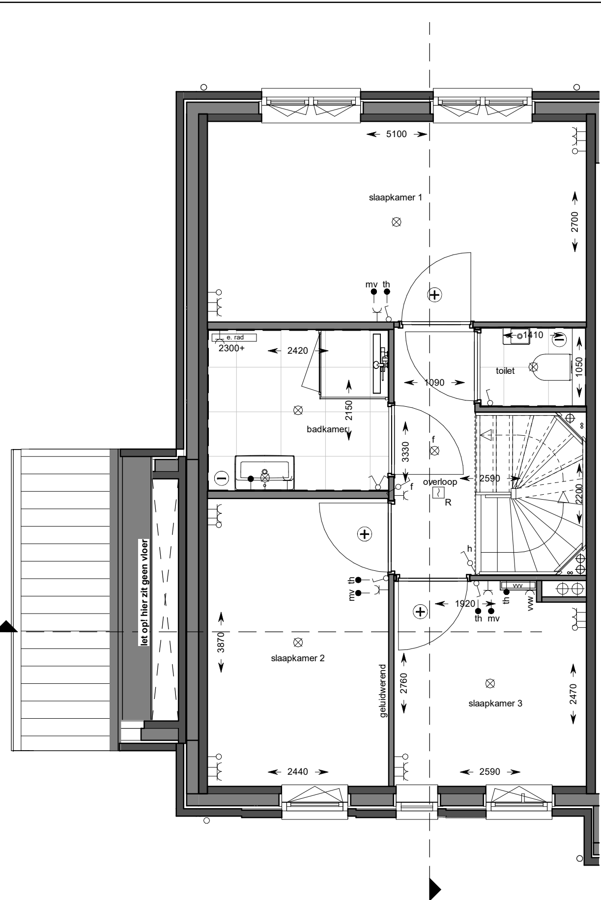
eerste verdieping
