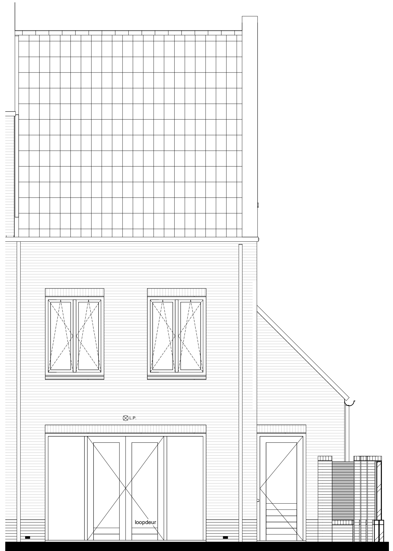
achtergevel
